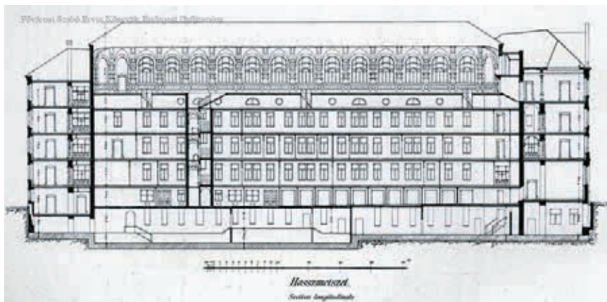
A telefonközpont épületének hosszmetSZete
